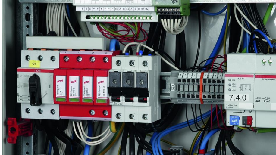
Imagem 1. DPS DEHN protegendo instalações elétricas.
